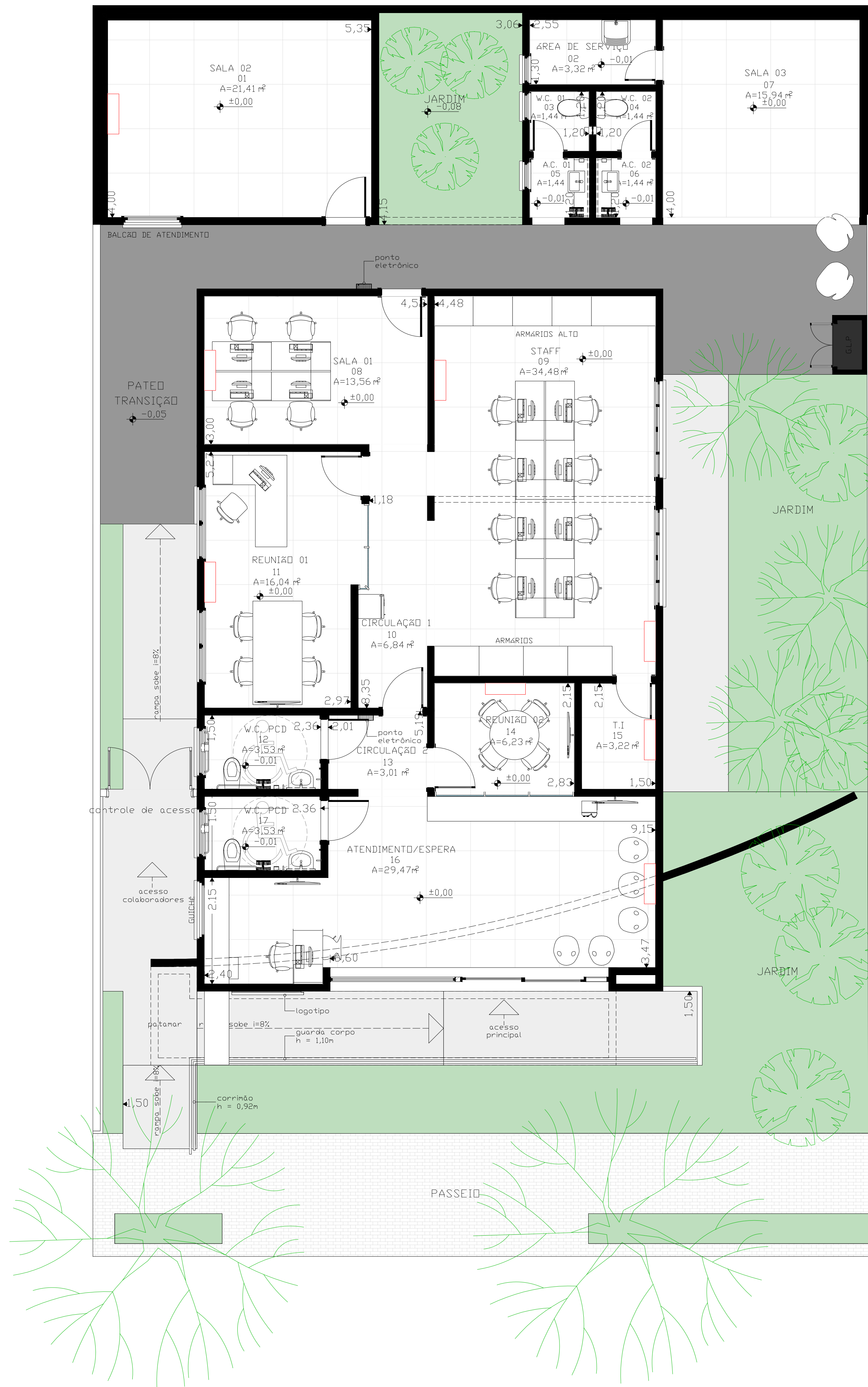
LAYOUT Escala: 1:50
