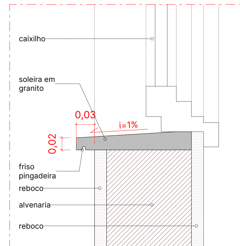
DETALHE ARQ 01 Escala: 1:3
