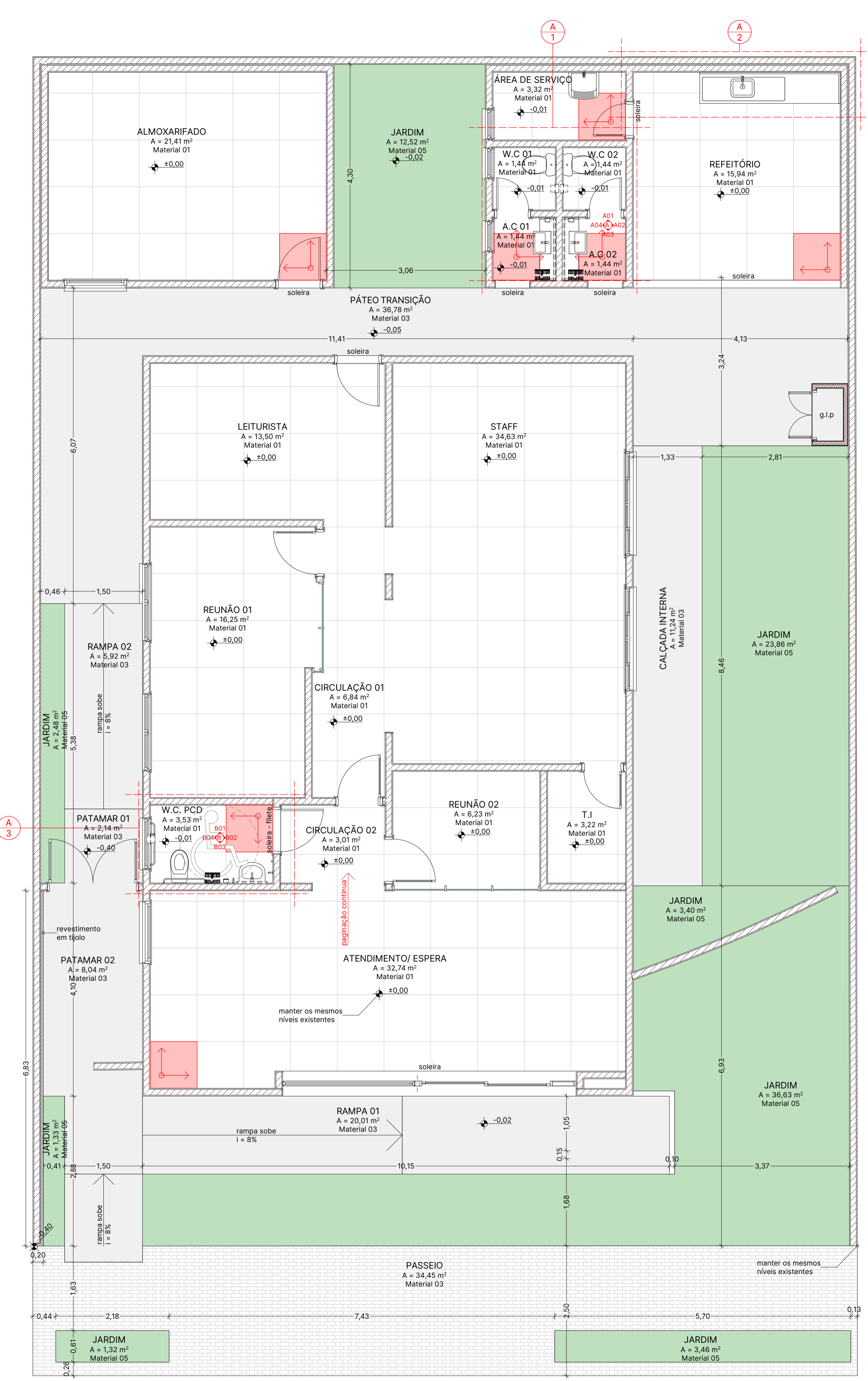
PAGINAÇÃO DE PISO Escala: 1:50
